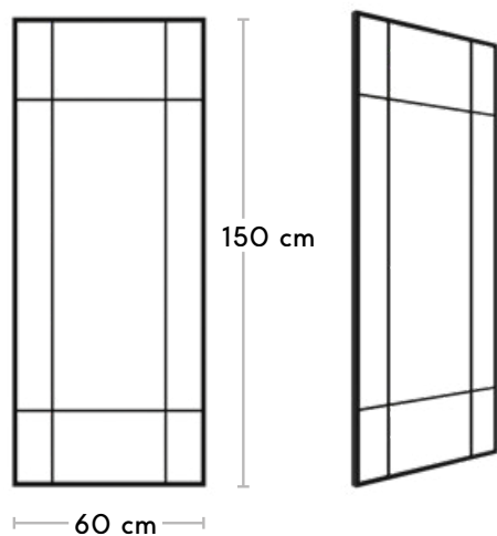
LFO5 • CONNOR • 60X150
