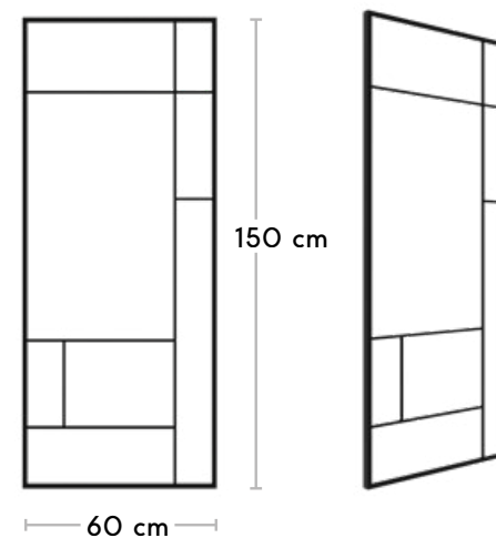
LFO6 • JACOB • 60X150
